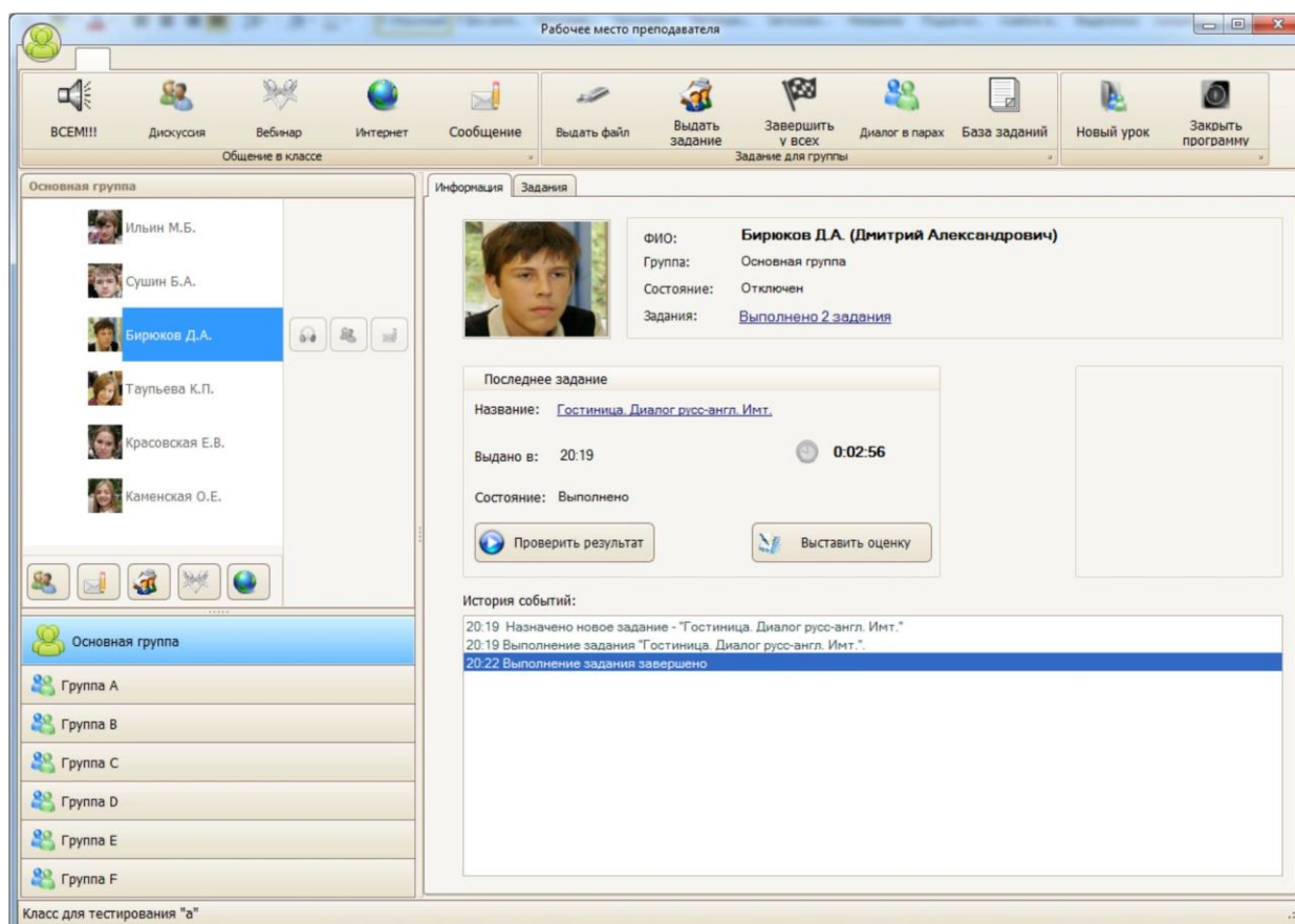
Рис. 1. Внешний вид интерфейса программы преподавателя
