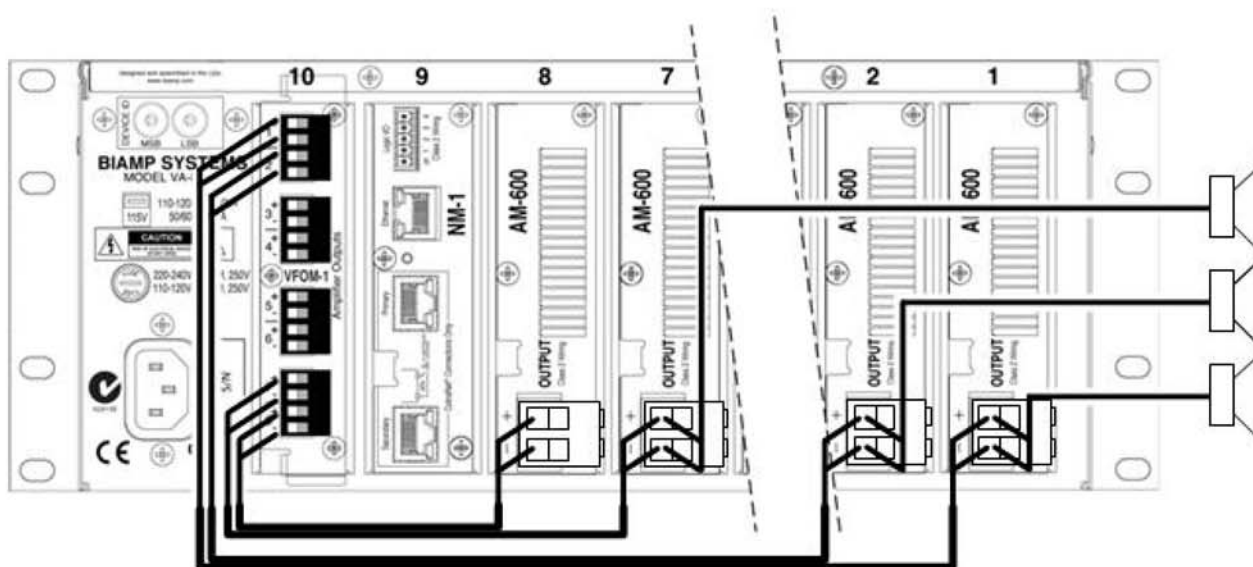
Резервирование канала 1 для работы вместо одного из каналов 2, 7, 8 в случае их неисправности
