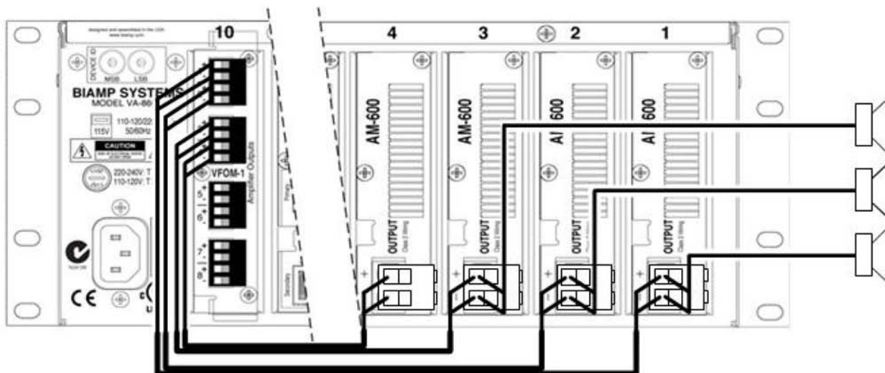
Резервирование канала 1 для работы вместо одного из каналов 2, 3, 4 в случае их неисправности
