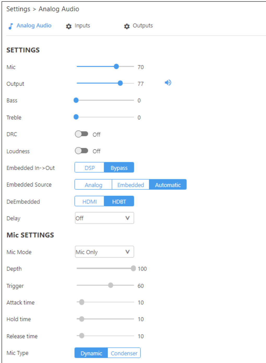
Figure 14: AV – Analog Audio Settings
