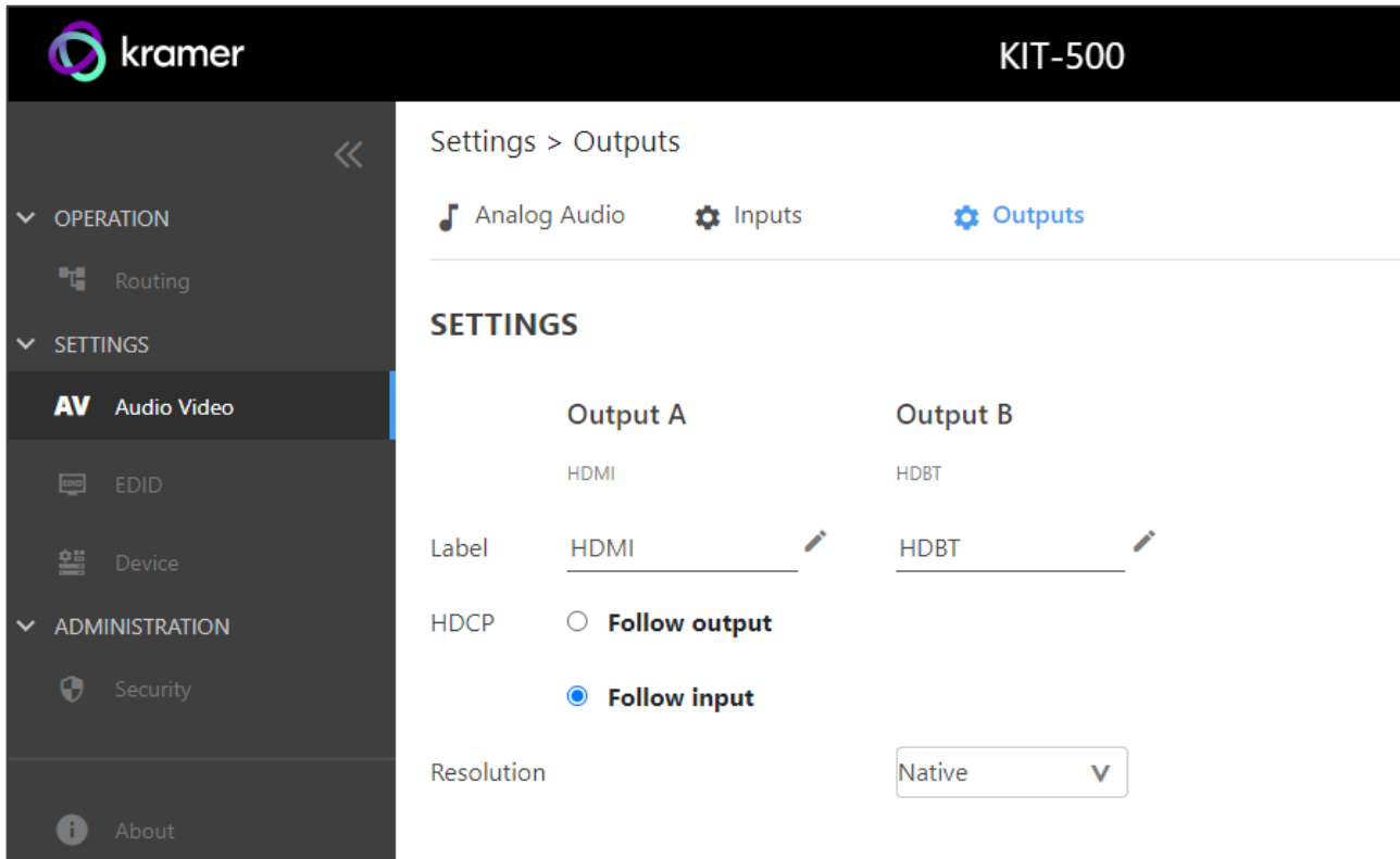
Figure 17: AV Settings – Outputs Tab
