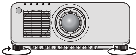
Максимальный диапазон настройки Регулируемые ножки: 30 мм (1-3/16") каждая
